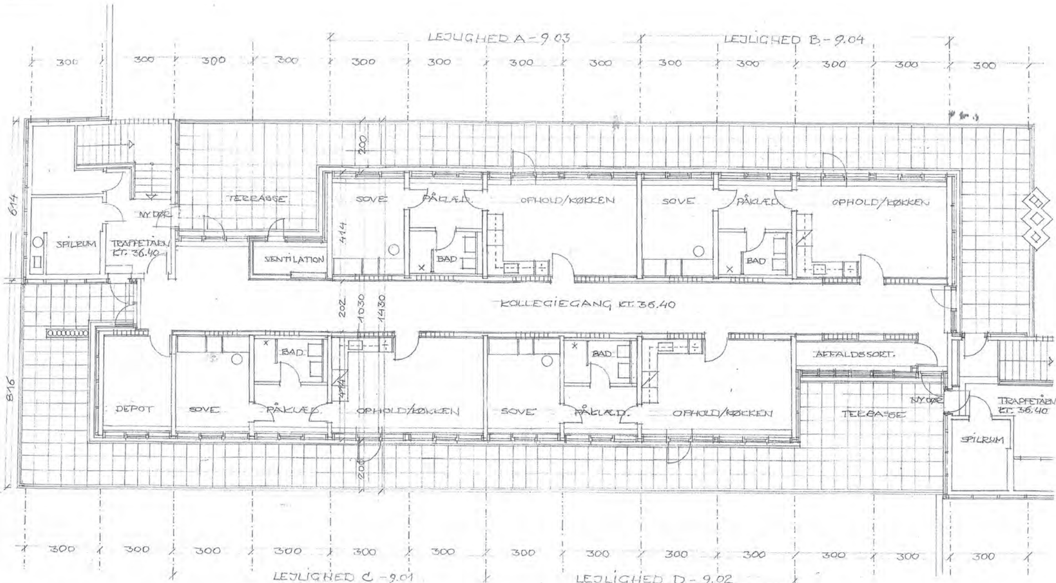
PLAN 9. ETAGE
